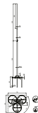
Maßbild
