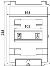
Maßbild IGA 6 IP54
