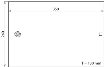
Maßbild DPG LSA 60 P
