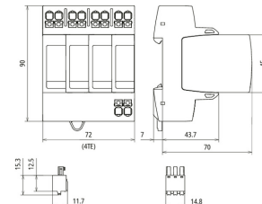
Maßbild DG MP TT ACI 275 FM
