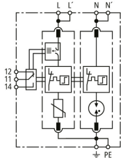
Prinzipschaltbild DG MP TN ACI 275 FM
