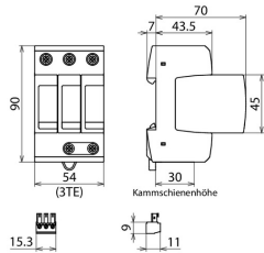
Maßbild DG M TNC ACI 275 FM
