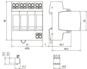
Maßbild DG SMP TNS 275 FM
