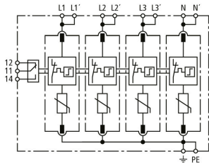
Principalschaltbild DG SMP TNS 275 FM
