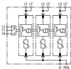
Prinzipschaltbild DG MP TNC 440 FM
