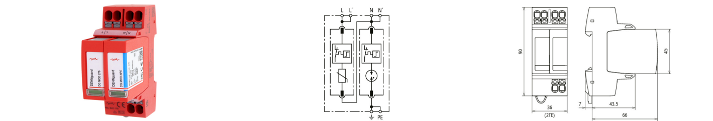
Abbildung unverbindlich Prinzipialschaltbild DG MP TT 2P 275 Maßbild DG MP TT 2P 275
