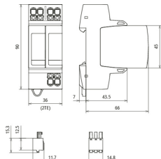
Maßbild DG MP TT 2P 320 FM
