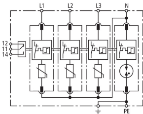
Prinzipschaltbild DG M TT 320 FM
