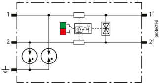
Prinzipschaltbild BCO ML2 BD HF 5
