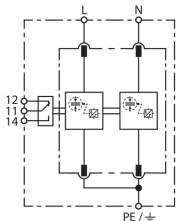
Prinzipschaltbild DV M2 TN 255 FM
