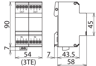
Maßbild
