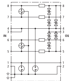
Prinzipschaltbild
