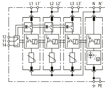
Prinzipschaltbild
