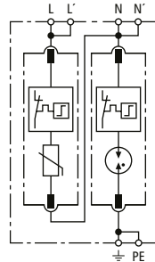
Prinzipschaltbild
