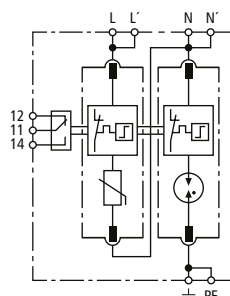
Prinzipschaltbild
