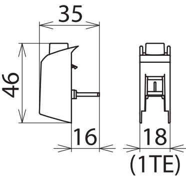
Maßbild
