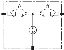
Prinzipschaltbild
