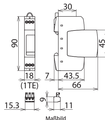
Maßbild
