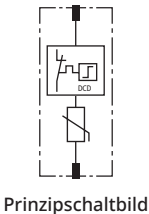
Prinzipschaltbild
