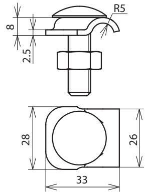
Maßbild KB 6.10 FRM10X35 CU
