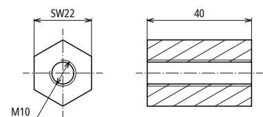
Maßbild DS SW22 M10 L40 V4A
