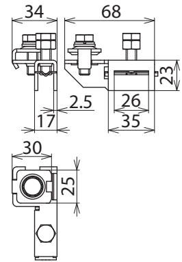
Maßbild SPK 27.89 BRS AK1X10 2X6.8 GSG
