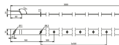
Maßbild AF 30X3.5 V4A ZW 3000
