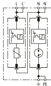
Prinzipialschaltbild DG MD TT 2P 275
