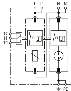
Prinzipschaltbild DG MD TT 2P 275 FM
