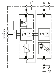
Prinzipialschaltbild DG MD TT 2P ACI 275 FM
