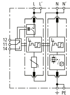
Prinzipschaltbild DG MD TT 2P ACI 385 FM
