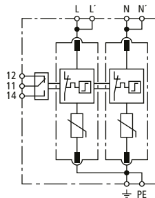
Prinzipschaltbild DG MD TN 275 FM
