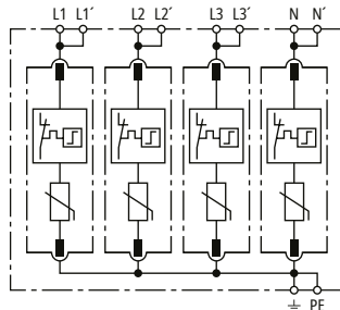
Prinzipialschaltbild DG SMD TNS 275
