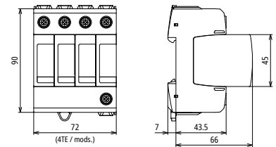
Maßbild DG SMD TNS 275
