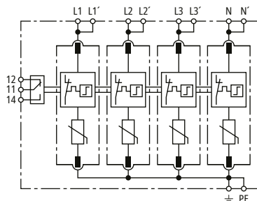
Prinzipialschaltbild DG SMD TNS 275 FM
