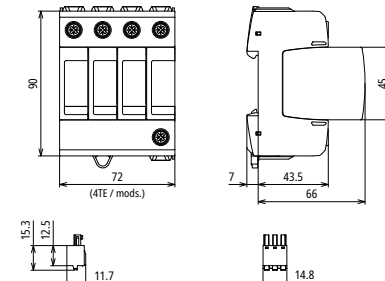
Maßbild DG SMD TNS 275 FM
