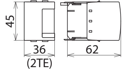
Maßbild DV MOD NPE 50
