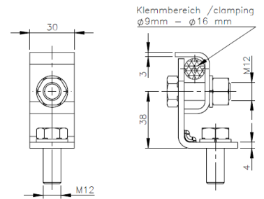
Maßbild SBKW PH3
