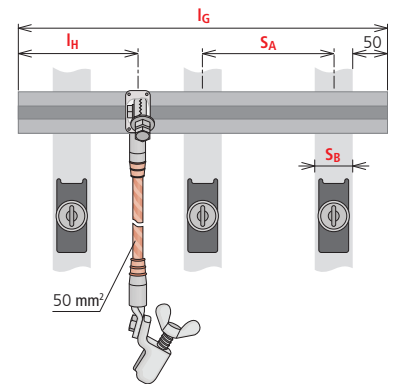
Maßbild KS SK A NS VP33XYL
