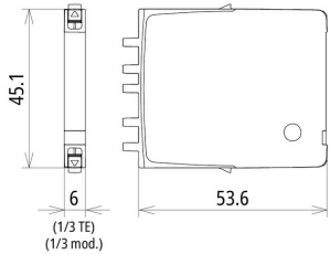
Maßbild BCO MOD ML2 B 180
