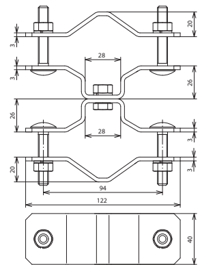
Maßbild BS D40.50 D48.60 V2A
