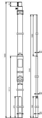
Maßbild SR D50 5000 FS2500 IP SA HVIP
