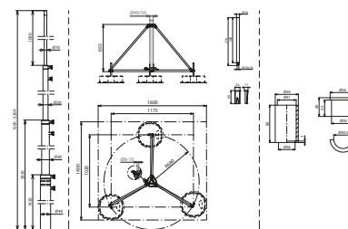
Maßbild FS T D40 1.5 5.2M AL DBS RA680
