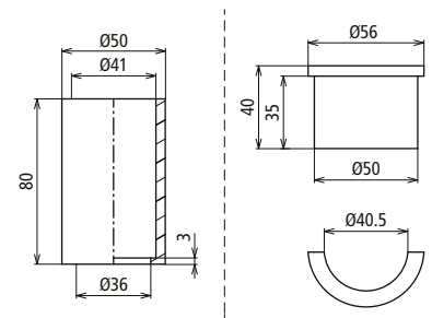
Maßbild RED D40 V2A DBS VBS
