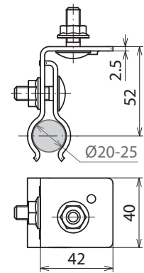
Maßbild HA M8 RSF20.25 V2A
