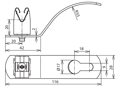
Maßbild DLH DQ 8 WPRO5 V2A STTZN
