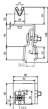
Maßbild DLH DG 8 KF18.22 AL
