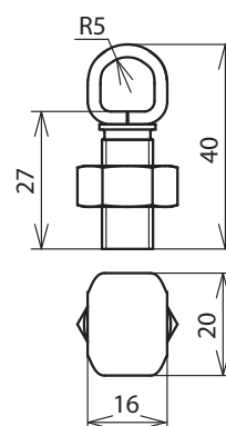
Maßbild KSV 8.12.5 CU
