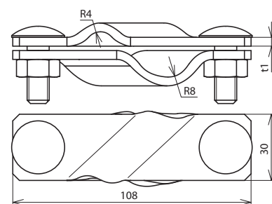
Maßbild SVK 7.10 16 FL40 STTZN
