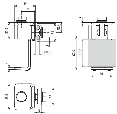
Maßbild AKK DUL 8.10 KBF 36 52 V2A
