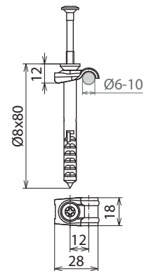
Maßbild LH DQ 6.10 ND8X80 STTZN
