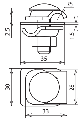
Maßbild ZMMVK 6.8 FRM10X35 CU STTZN
