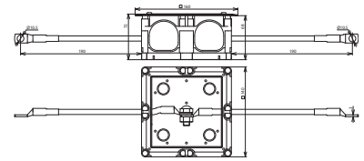
Maßbild TSK 140X140 V2A AL16CU
