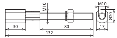
Maßbild GAD EFP M10 10 L130 V4A
